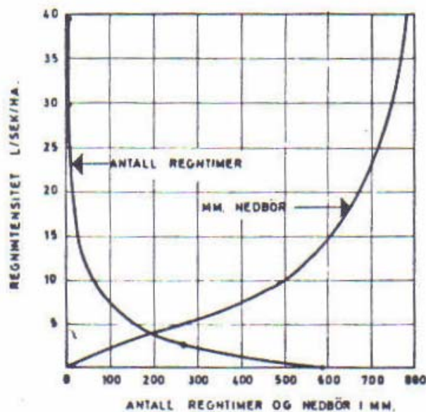
FIG. 10.3. VARIGHETSKURVE FOR INTENSITETEN, OG DE FORSKJELIGE INTENSITETERS BIDRAG TIL DEN SAMLEDE ARSNEDBÖR. PLUVIOGRAFMALINGER PÅ BRYNE, TIME KOMMUNE I TIDEN 26-6-65 - 20-6-66.
