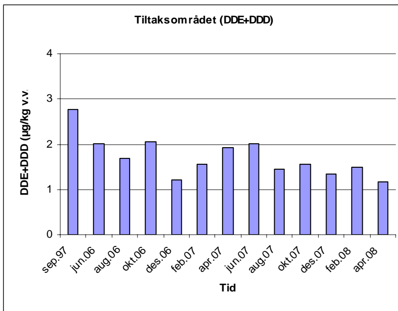
Figur 10. Summen av DDE og DDE, mudringsområdet. DDE og DDD inngår ikke i SFTs klassifiseringssystem.
