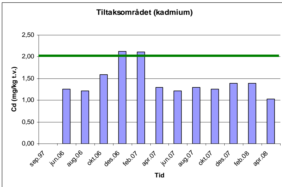
Figur 3. Kadmium (Cd), tiltaks-/mudringsområdet. Under grønn strek: Kl. I, Ubetydelig/lite forurenset Over grønn strek: Kl. II, Moderat forurenset
