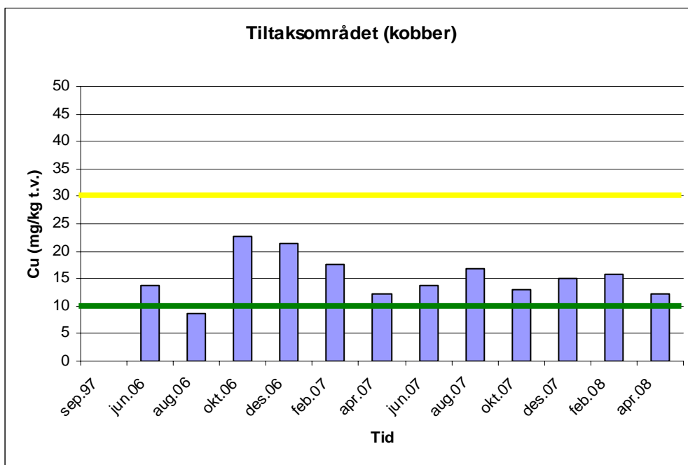
Figur 4. Kobber (Cu), tiltaks-/mudringsområdet. Under grønn strek: Kl. I, Ubetydelig/lite forurenset Over grønn strek/under gul strek: Kl. II, Moderat forurenset Over gul strek: Kl. III, Markert forurenset
