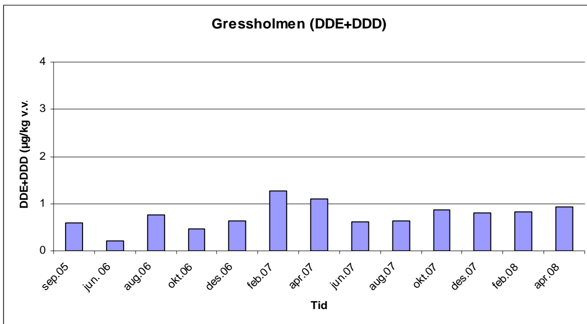
Figur 22. DDE+DDD, Gressholmen. Forbindelsene inngår ikke i SFTs klassifiseringssystem.
