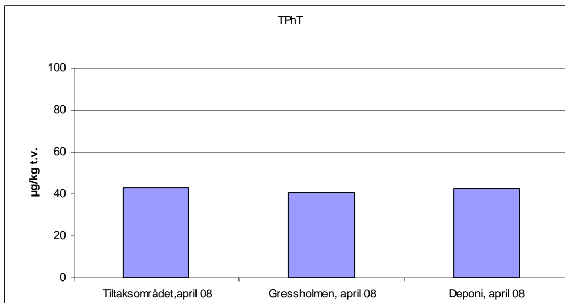
Figur 46. TPhT i skjell fra tiltaks-/mudringsområdet, Gressholmen og deponiområdet i april 2008.
