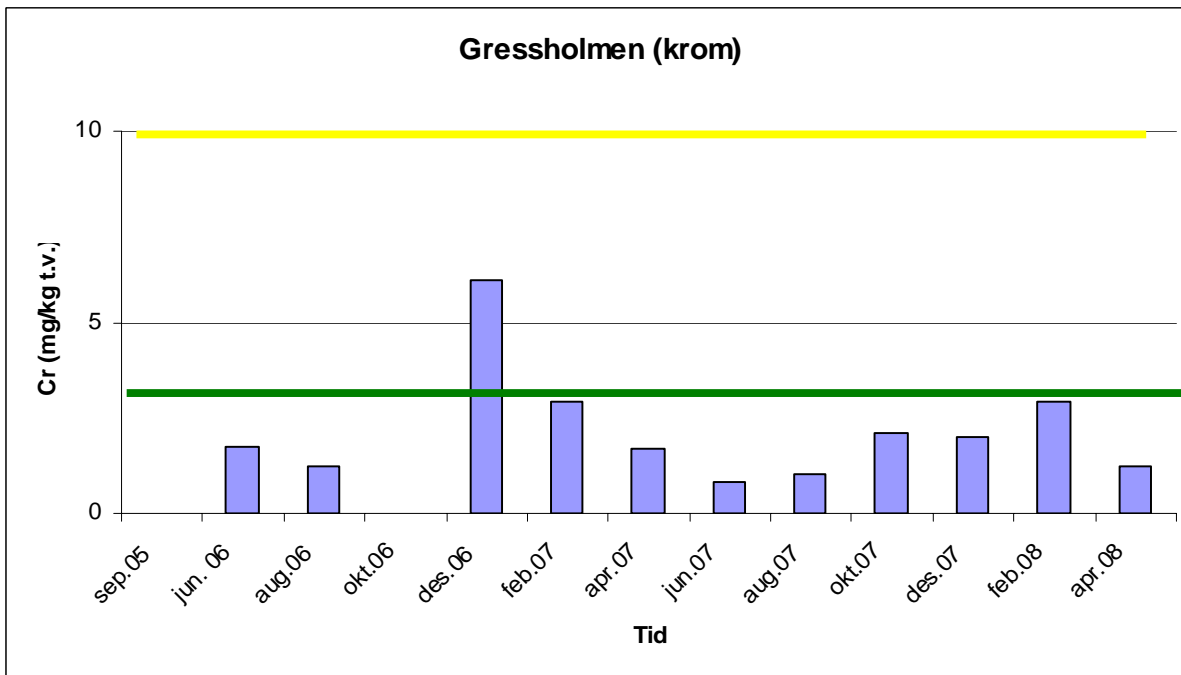
Figur 20. Krom (Cr), Gressholmen.
