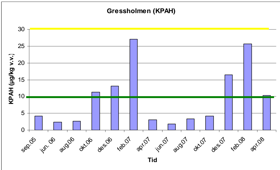
Figur 24. Sum KPAH, Gressholmen.
