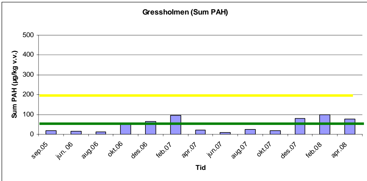
Figur 23. Sum PAH, Gressholmen.
