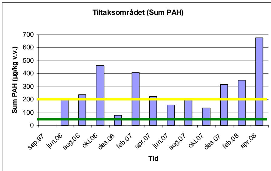
Figur 11. Sum PAH, tiltaks-/mudringsområdet.
