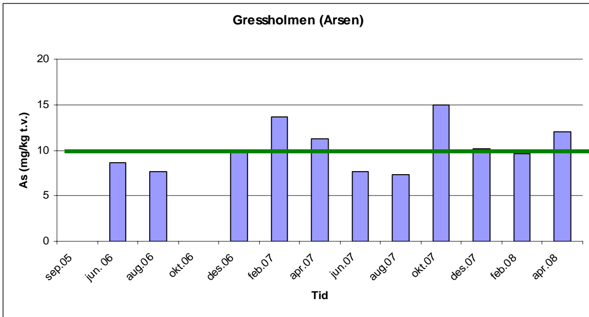
Figur 19. Arsen (As), Gressholmen.
